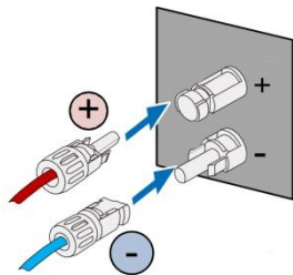
图 5.4 光伏直流组串接入逆变器
