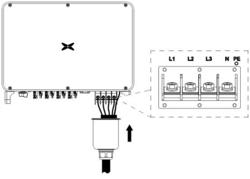
图 5.8 三相逆变器电网接入
