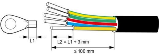
图 5.7 压接电缆端子
