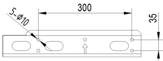
图 4.6 安装挂板尺寸图
