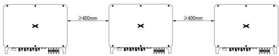
图 4.5 并排安装尺寸要求
