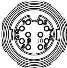
图 5.6 DRM & RS485 端子正视图
