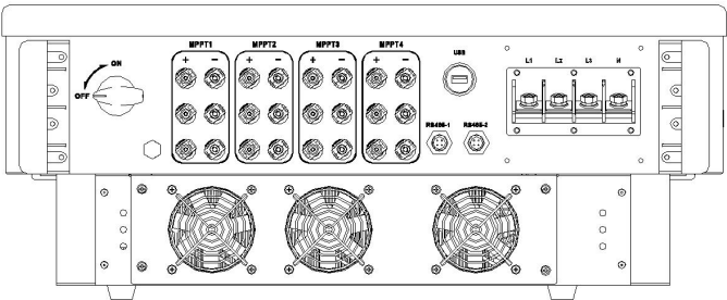
50kWR 底部视图
